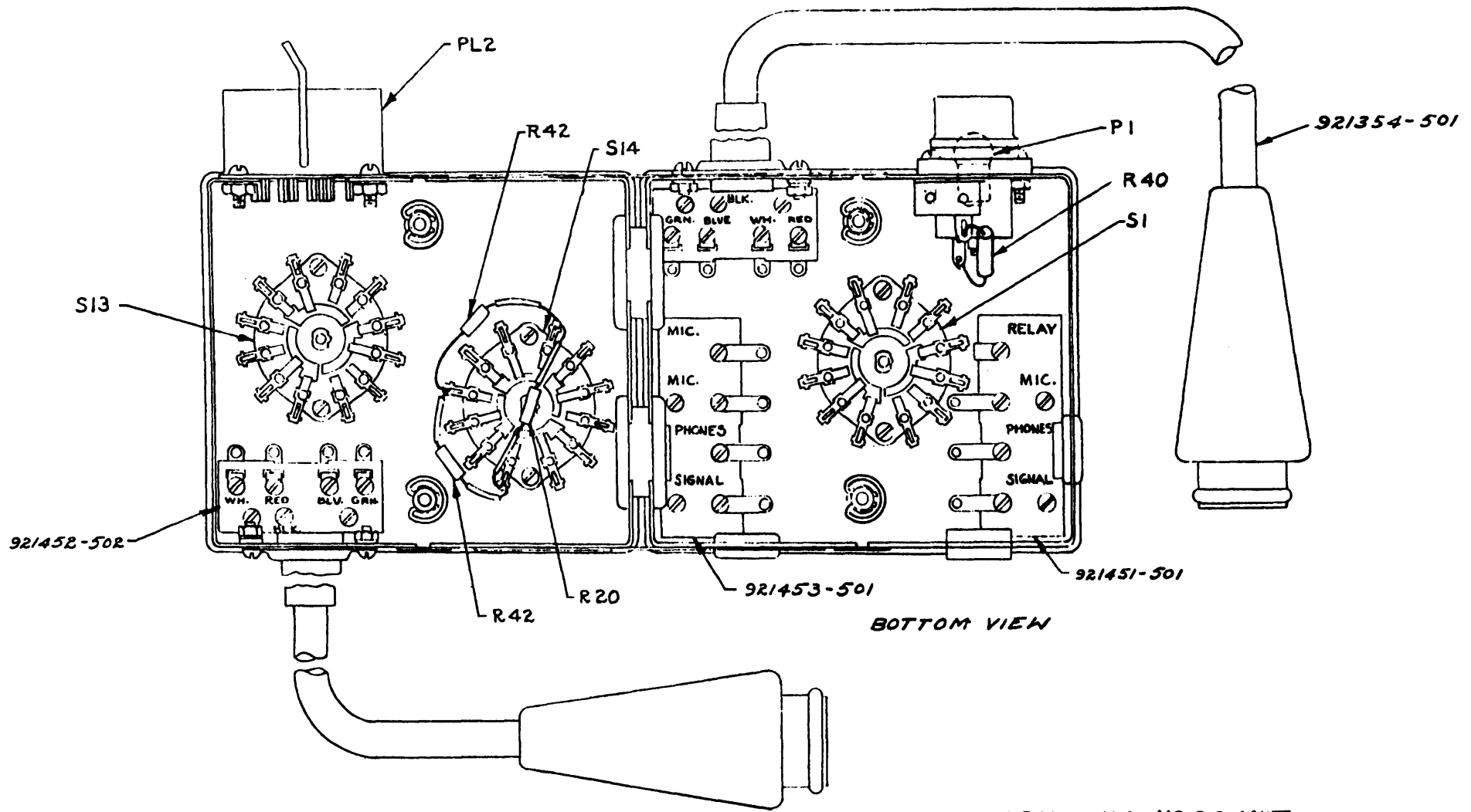
CONTROL UNIT NR 3C MKII
